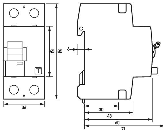
Dibujo acotado DFS 2 A HD, 2 polos (Vista de grupos)
