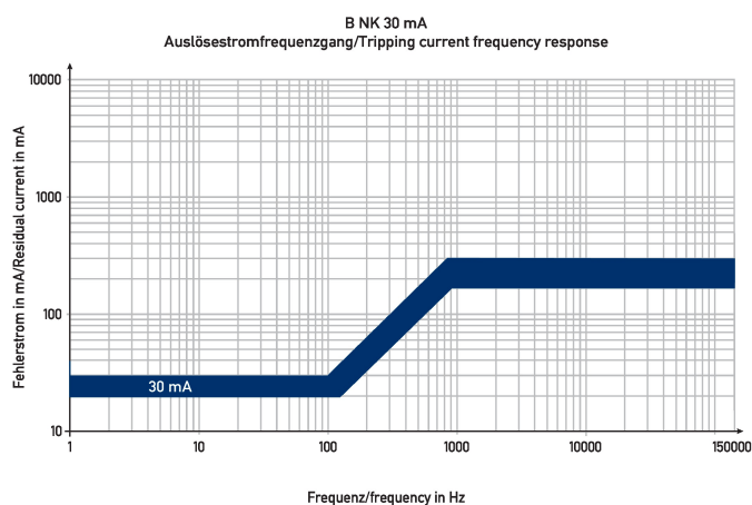
Curva característica B NK 30 mA
