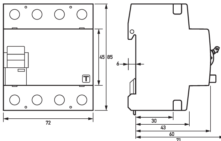
Dibujo acotado DFS 4 B NK V500, 4 polos (Vista de grupos)
