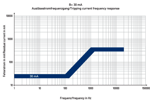
Diagramme Fehlerstromschutzschalter DFS 4 016-4/0,03-B+ HD
