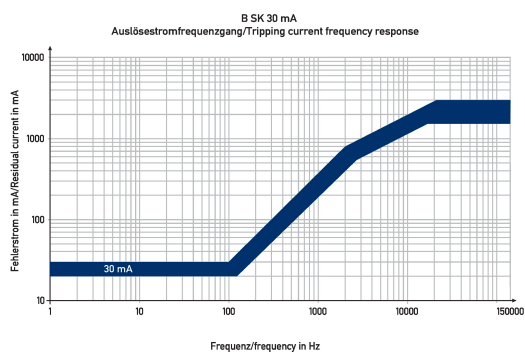
Diagramme Fehlerstromschutzschalter DFS 4 016-4/0,03-B SK MI HD
