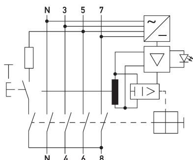
Schaltungsbeispiel Fehlerstromschutzschalter DFS 4 016-4/0,03-B SK MI HD
