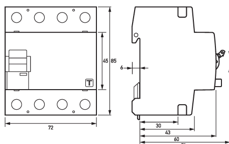
Maßzeichnung Fehlerstromschutzschalter DFS 4 016-4/0,03-B SK MI HD
