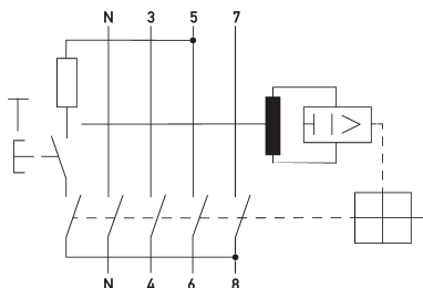
Esquema de conexiones
