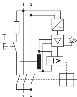
Esquema de conexiones DFS 2 B SK Hz, 2 polos
