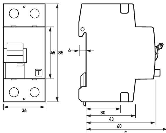
Dibujo acotado DFS 2 B SK Hz, 2 polos (Vista de grupos)
