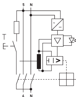
Esquema de conexiones DFS 4 B SK V, 2 polos
