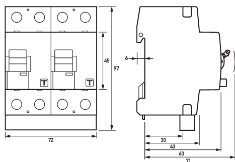
Maßzeichnung Fehlerstromschutzschalter DFS 2 016-2/0,03-A KV Twin
