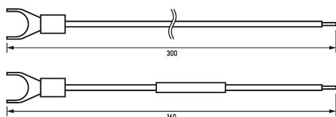
Dibujo acotado Cables DFA 2 - RC 100
