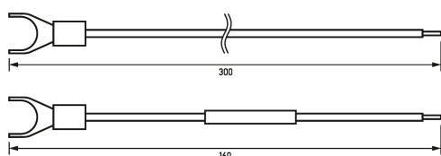
Dibujo acotado Cables DFA 2 - RC 030
