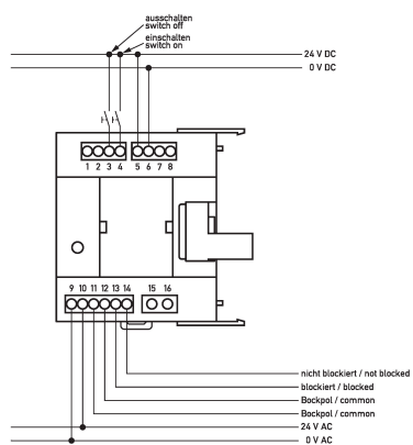
Anschlussschema
