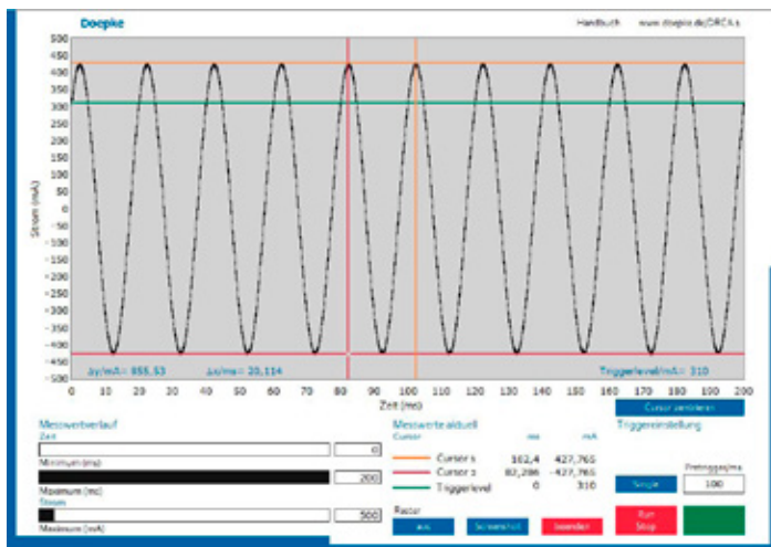
Abb. 9: Triggermodus
