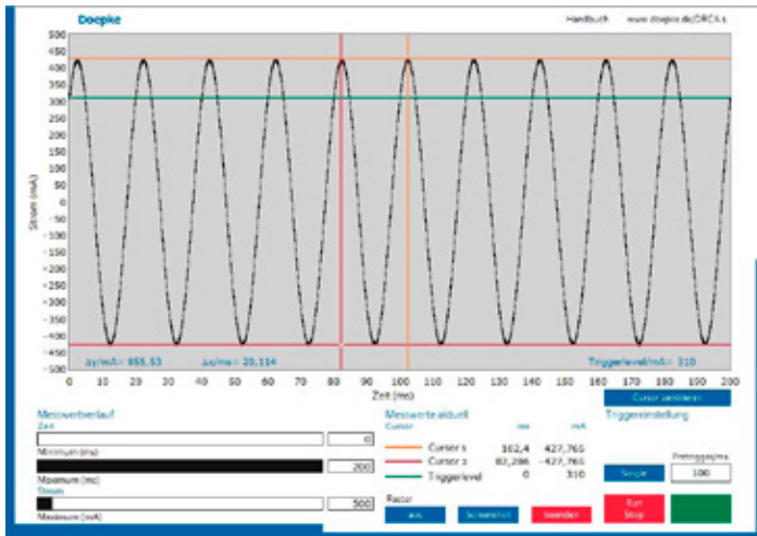
Abb. 9: Triggermodus
