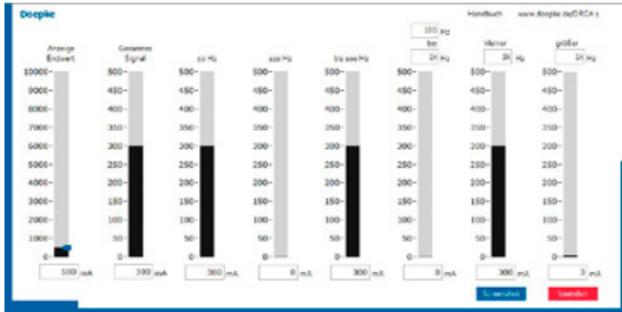
Abb. 5: Effektivwertanzeige
