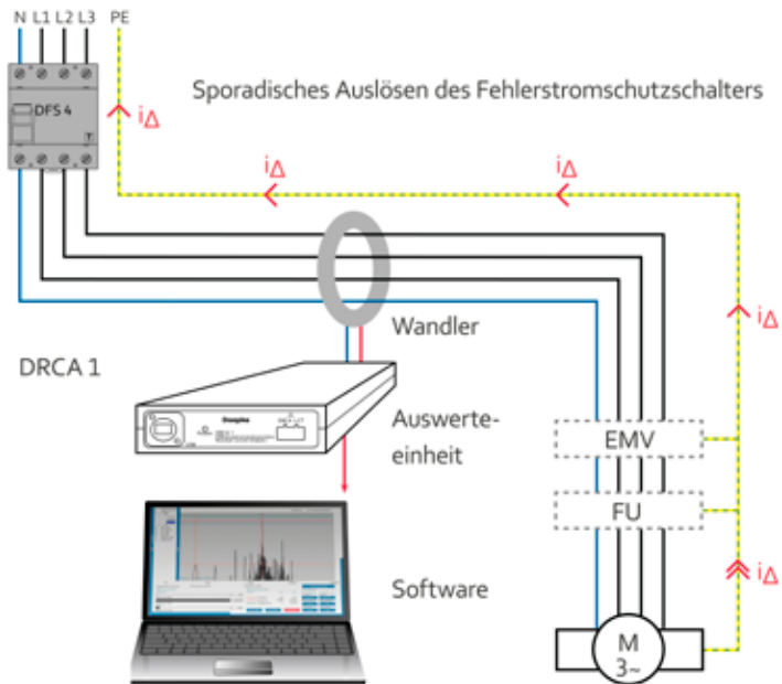
Abb. 1: schematischer Aufbau des Messsystems
