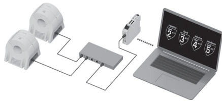
▲ Anschlussschema e.Guard RCM, PoE-Switch und e.Guard-Gateway in Level 2.
