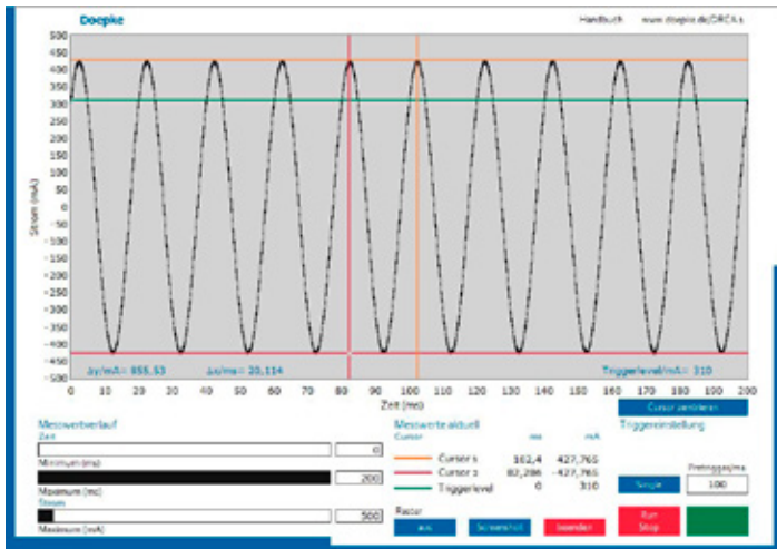
Abb. 9: Triggermodus
