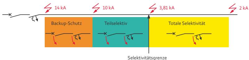
Abb. 18: Darstellung Teilselektivität
