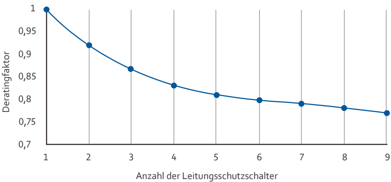
Abb. 24: Derating aneinander gereichte LS
