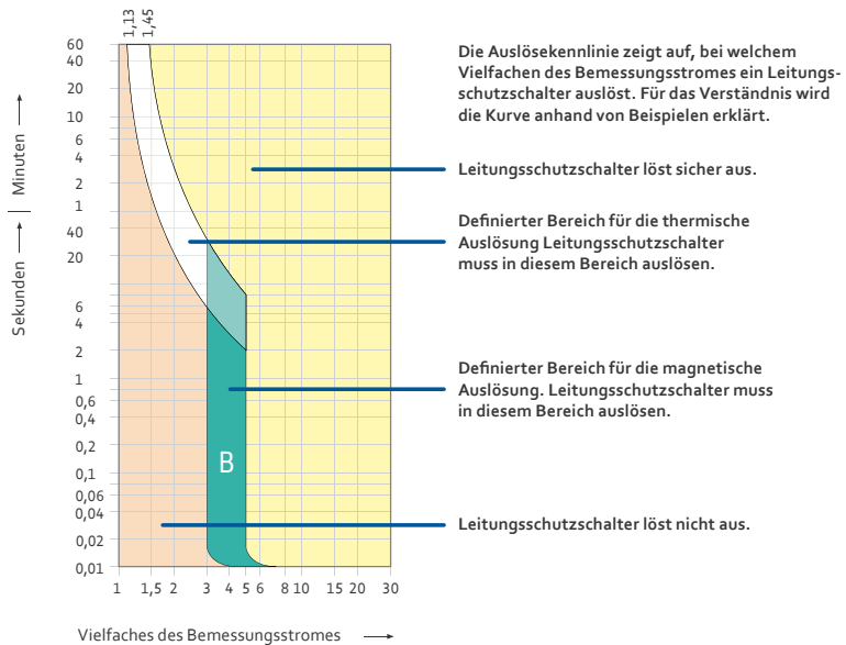
Abb. 6: Auslösekurve B-Charakteristik
