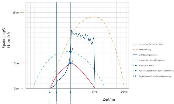
Abb. 11: Schematische Darstellung des strombegrenzenden Abschaltes | Strom- und Spannungsverlauf
