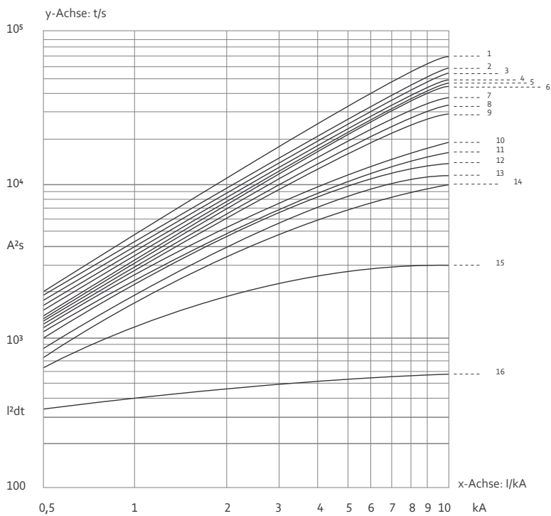
Abb. 21: Durchlasskennlinien C-Charakteristik
