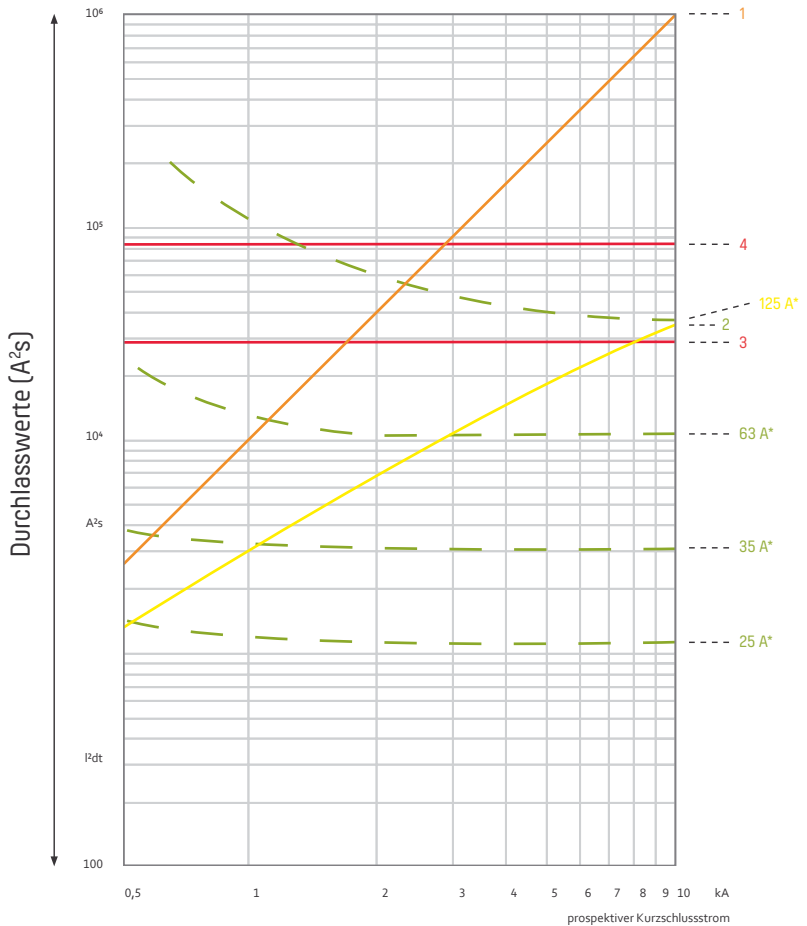
Abb. 16: Durchlassenergie
