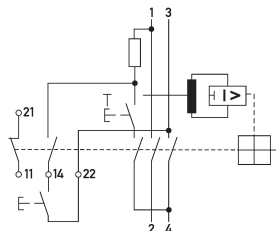
Esquema de conexiones
