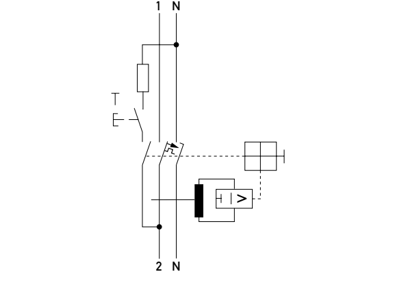
Schaltbild
