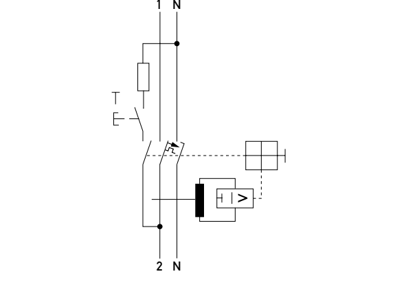
Schéma zapojení
