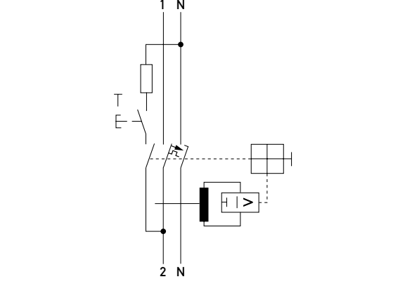
Schéma zapojenia
