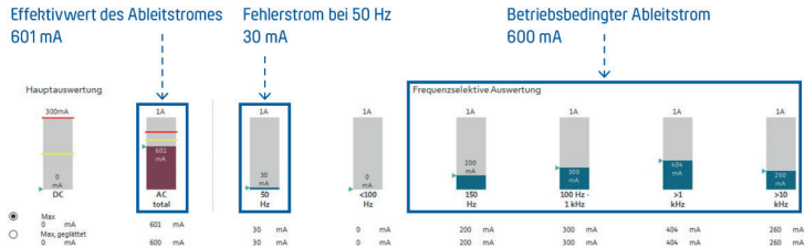
Abb. 15: Frequenzselektive Auswertung der Differenzströme mit e.Guard RCM B und Zuordnung der einzelnen Frequenzen
