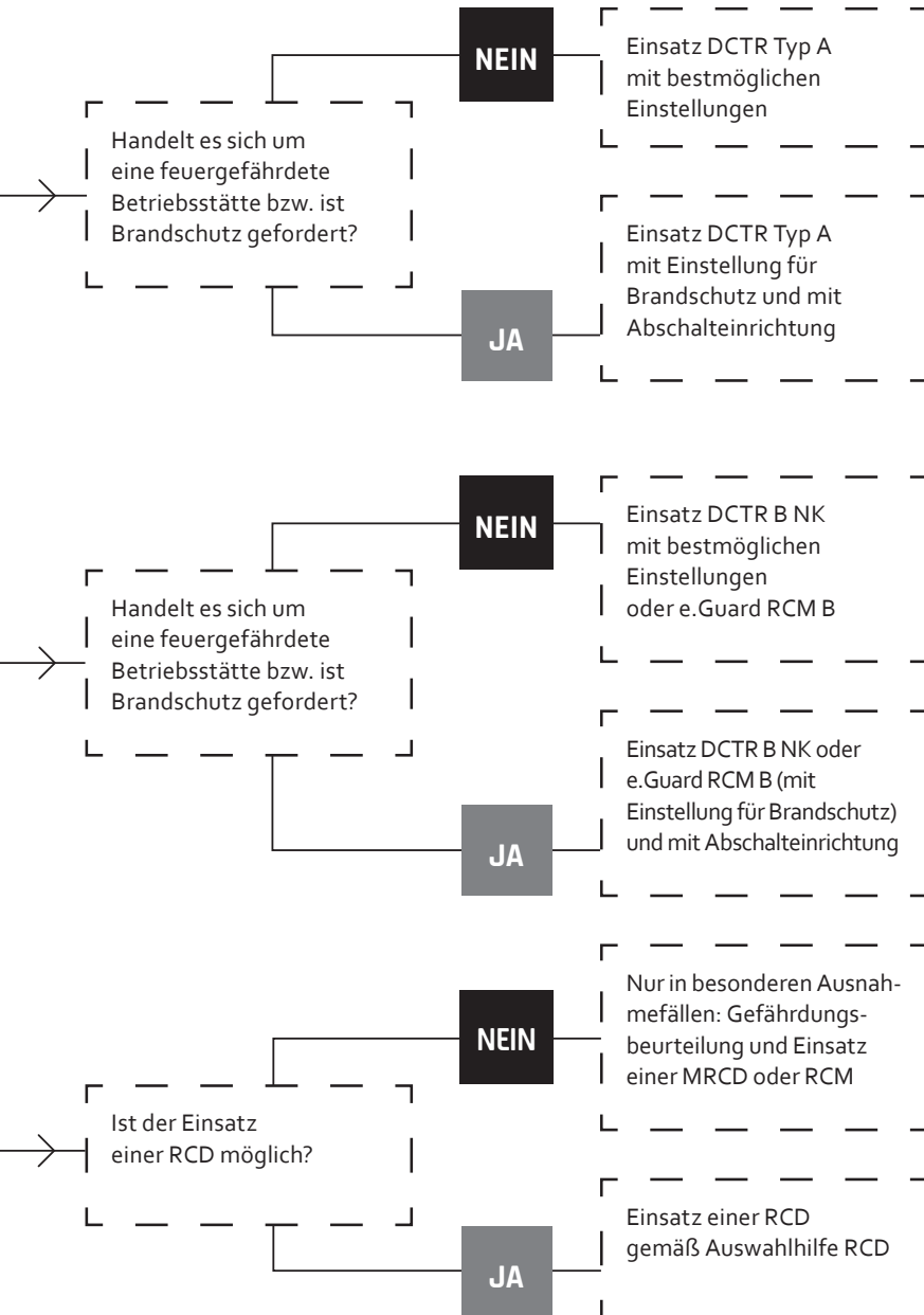
Abb. 26: Auswahlhilfe RCM-Systeme
