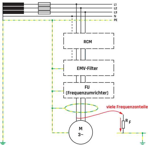
Abb. 6: Fehlerstrom mit Frequenzgemisch
