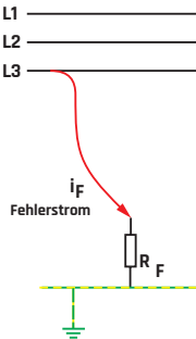
Abb. 2: Wechselfehlerstrom
