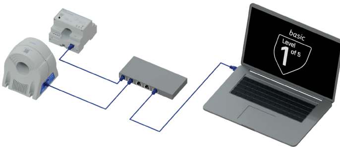
Abb. 20: Aufbau e.Guard basic
