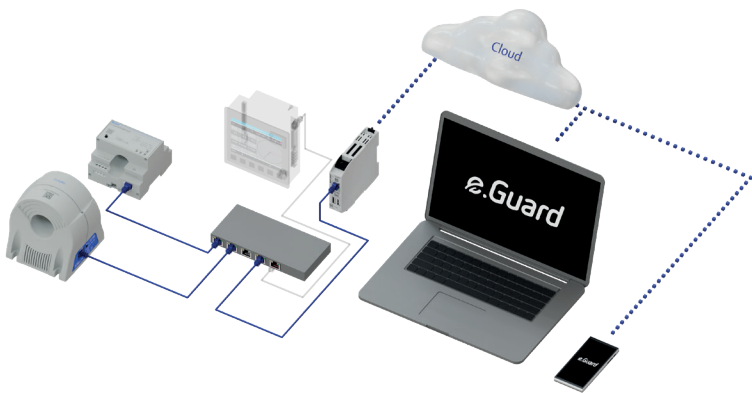
Abb. 19: Aufbau e.Guard RCM mit Netzwerkswitch und e.Guard Gateway
