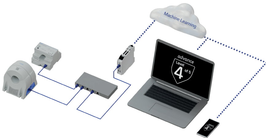
Abb. 23: Aufbau e.Guard advance
