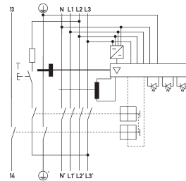
Anschlusschema
