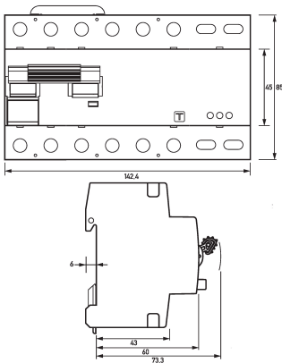
Maßzeichnung Gruppenansicht
